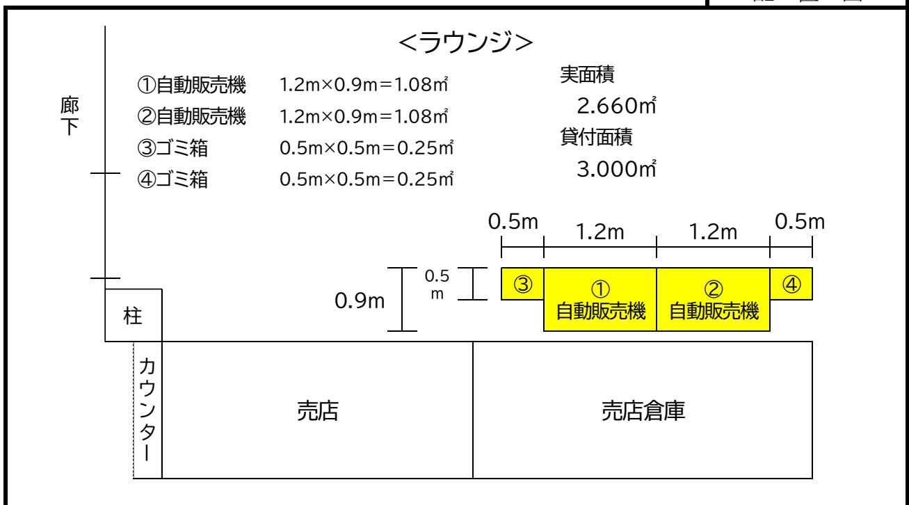
配置図
