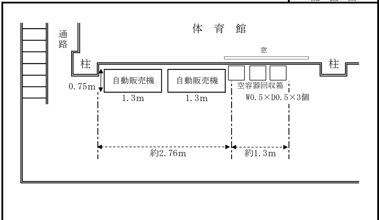
配 置 図
