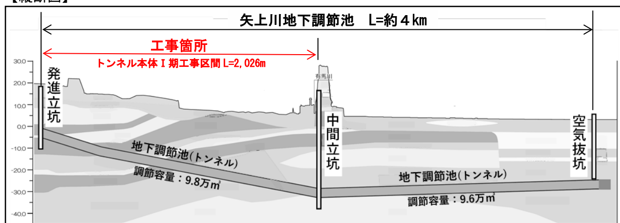
【縦断図】
