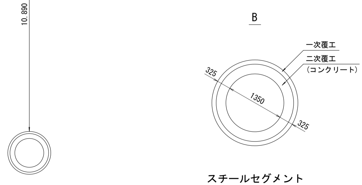
管渠構造図 S=1:50
