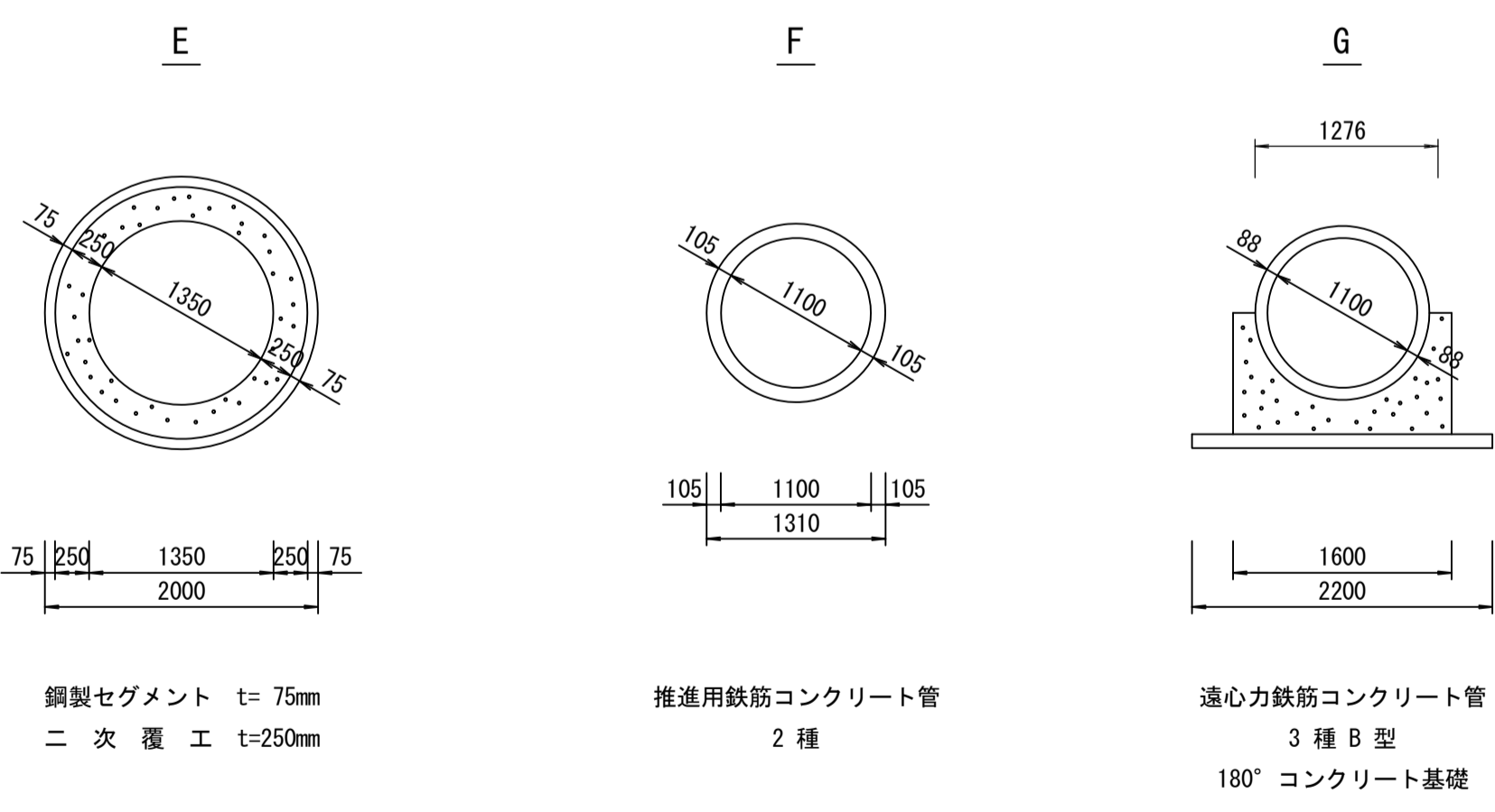
管渠構造図 S=1:50
