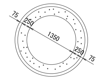
鋼製セグメント t=75mm 二次覆工 t=250mm
