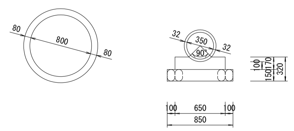
推進用鉄筋コンクリート管 鉄筋コンクリート管 外圧管 2種 B型
