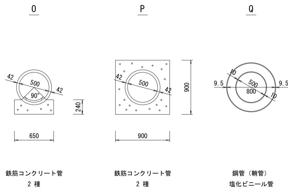
管渠構造図 S=1:30
