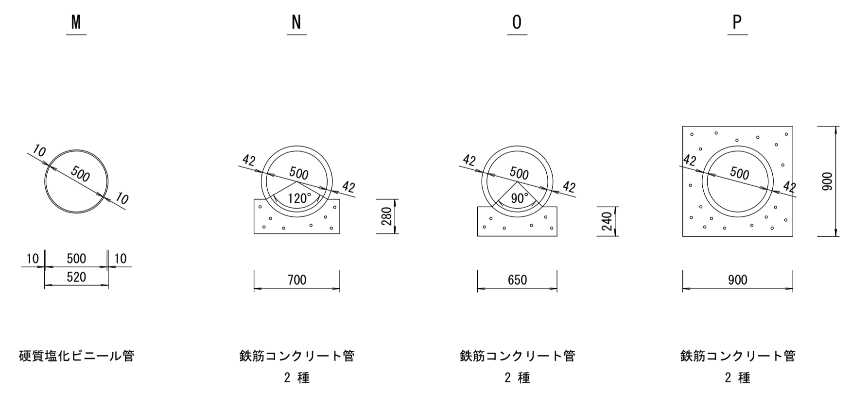
管渠構造図 S=1:30
