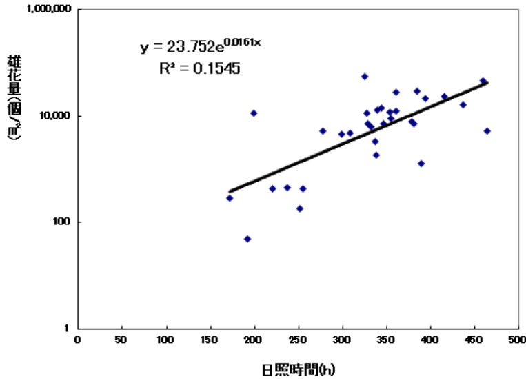
図4 7月・8月の日照時間とヒノキ雄花量(小田原市久野)の関係
