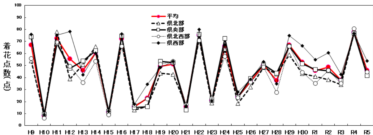
図1 スギ地域別の着花点数の年変化
