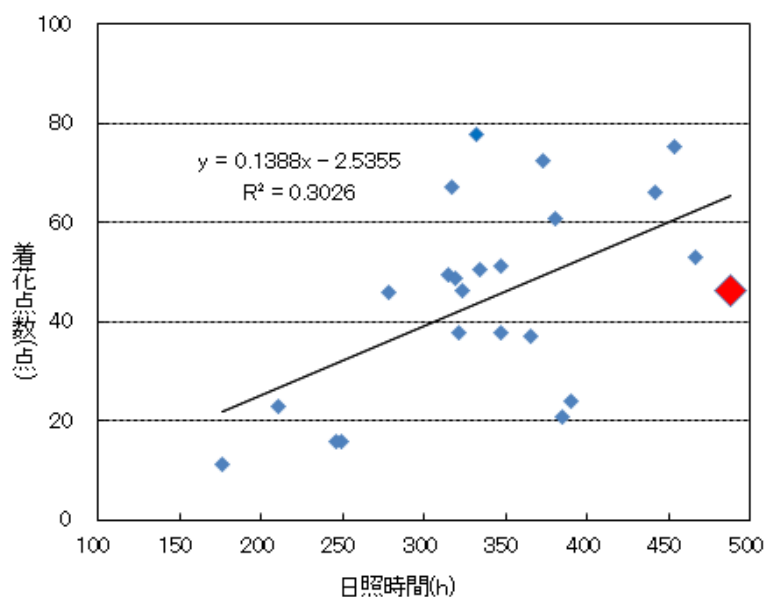
図3 7月・8月の日照時間とスギ着花点数の関係
