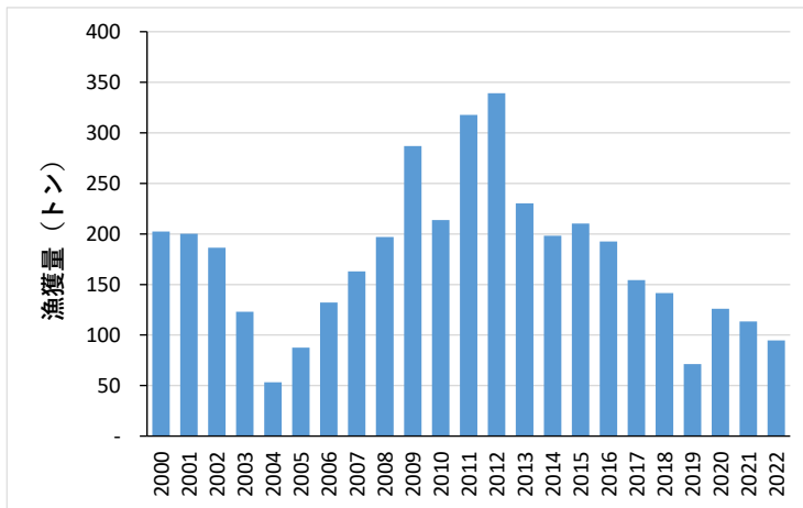
アカカマス漁獲量の経年変化 ※神奈川県定置網漁海況調査表より
