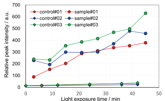
図5 ESR測定結果 (controlは、TiO 2 なし光照射の比較)
