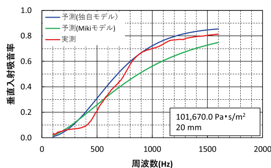
図1 グラスウール(平均繊維径 3\mu\text{m} )の垂直入射吸音率の比較
