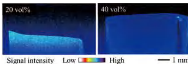
図5 固体含有率が異なる分散系スラリーの乾燥体のOCT像
