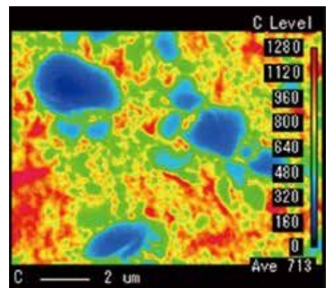
正極のEPMA分析
