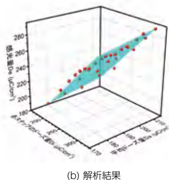
図1 8ステップパターンの各ステップのドーズ量 D_i 、パターンの平均ドーズ量 D_0 と感光ドーズ量 D_0 の関係
