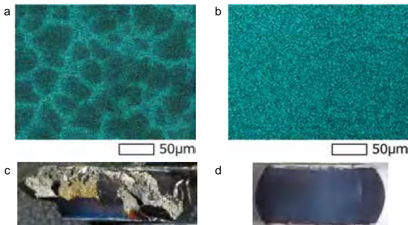
Cuに関するSEM-EDS結果と圧縮試験後の試料写真 (a, c: 鑄造まま材, b, d: 熱処理材)
