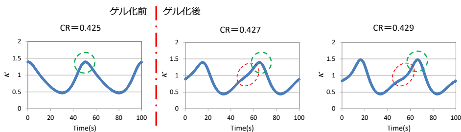
図3 \kappa の1周期変化（ \gamma_0=500\% 、 f=0.01 Hz）
