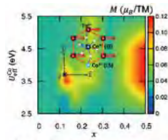
図2：理論的に解明したBiFe 1-x Co x O 3 の自発磁化の組成・電子相関依存性
