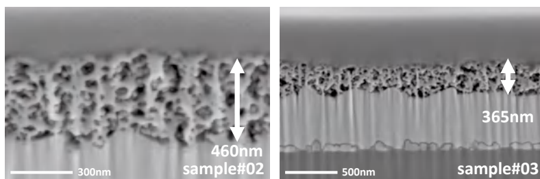
図3 sample#02の断面SEM像
