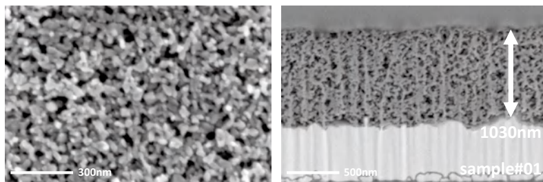
図1 TiO 2 の表面SEM (粒子径 約30nm)
