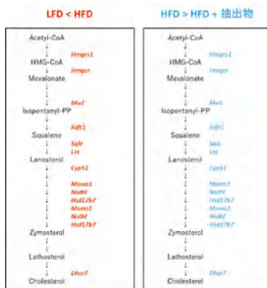
図3 コレステロール合成経路の変化 肝臓トランスクリプトーム解析より、左：低脂肪食(LFD)摂取群に対して高脂肪食(HFD)摂取群で発現増加した遺伝子を赤、右：高脂肪食(HFD)摂取群に対してナンノクロロプシス抽出物(HFD+抽出物)摂取群で発現減少した遺伝子を青で示した。
