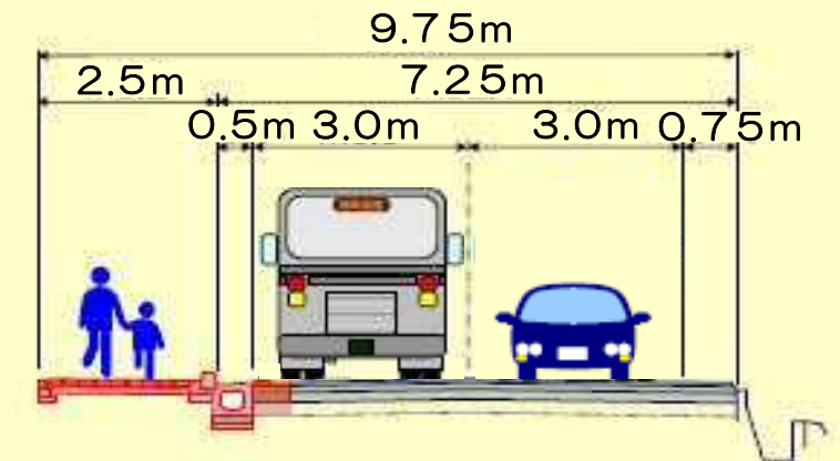
完成横断面図
