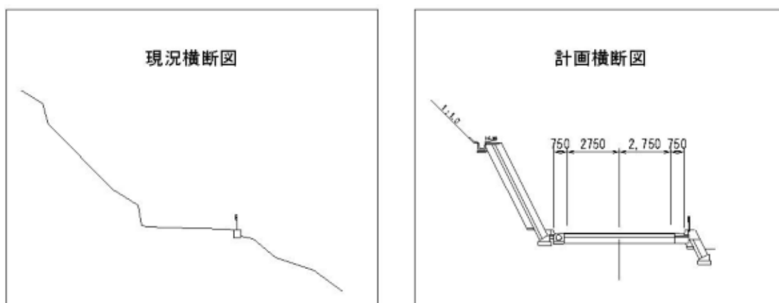
図:横断面図(単位:m)
