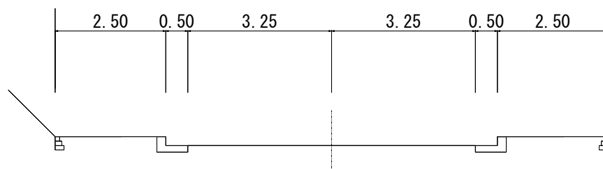
図：計画横断面図(単位:m)
