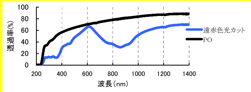
遠赤色光カットフィルムとPOフィルムの波長別光透過率
