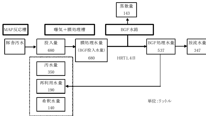
図1 各処理施設の水フロー(1/2再利用試験)
