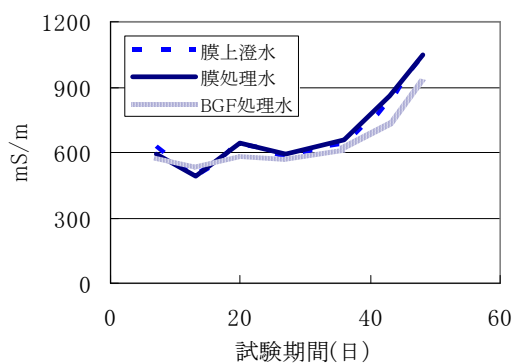
図2 全量再利用試験のECの推移
