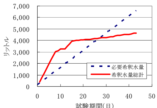
図3 必要希釈水量と希釈水量の推移
